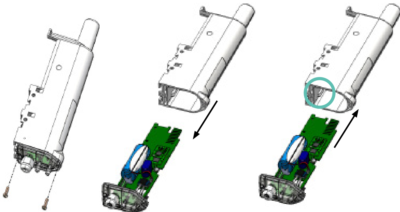
Tirer sur le presse-étoupe pour décoller la semelle
